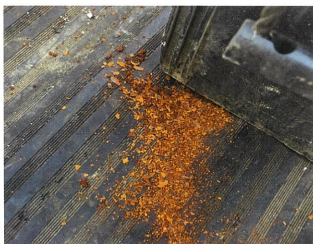
錆による冷却回路が詰まりオーバーヒートが発生した Daimler エンジン
